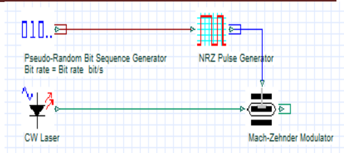
Fig. 2: NRZ Encoder
