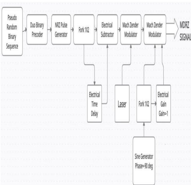
Fig. 1: MDRZ Encoder
