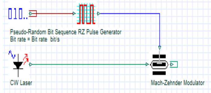
Fig. 3: RZ Encoder
